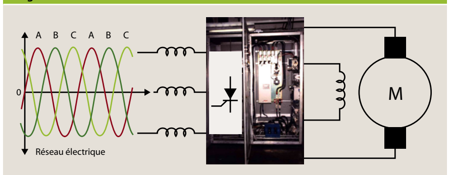
Figure 1 : Variateur de vitesse à courant continu
