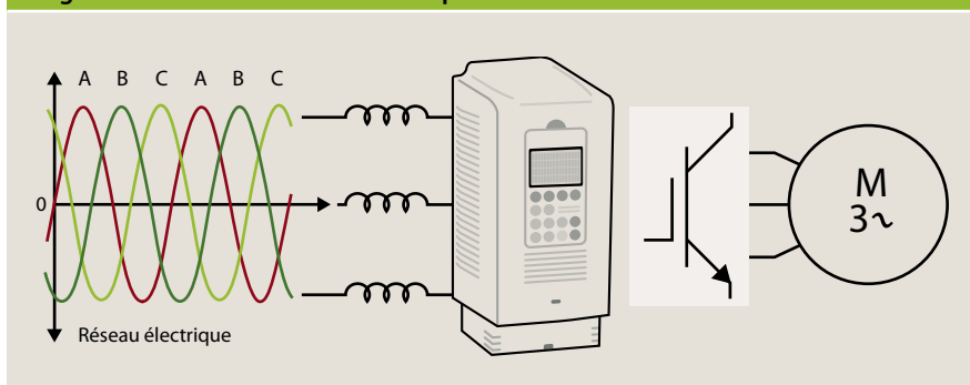
Figure 2 : Variateur de vitesse à fréquence variable
