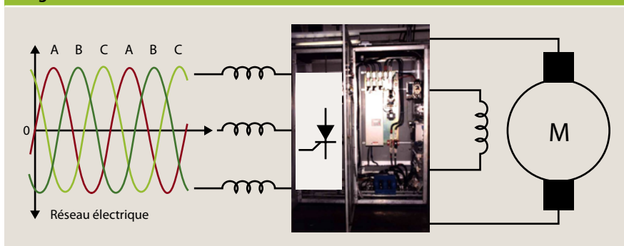
Figure 1 : Variateur de vitesse à courant continu
