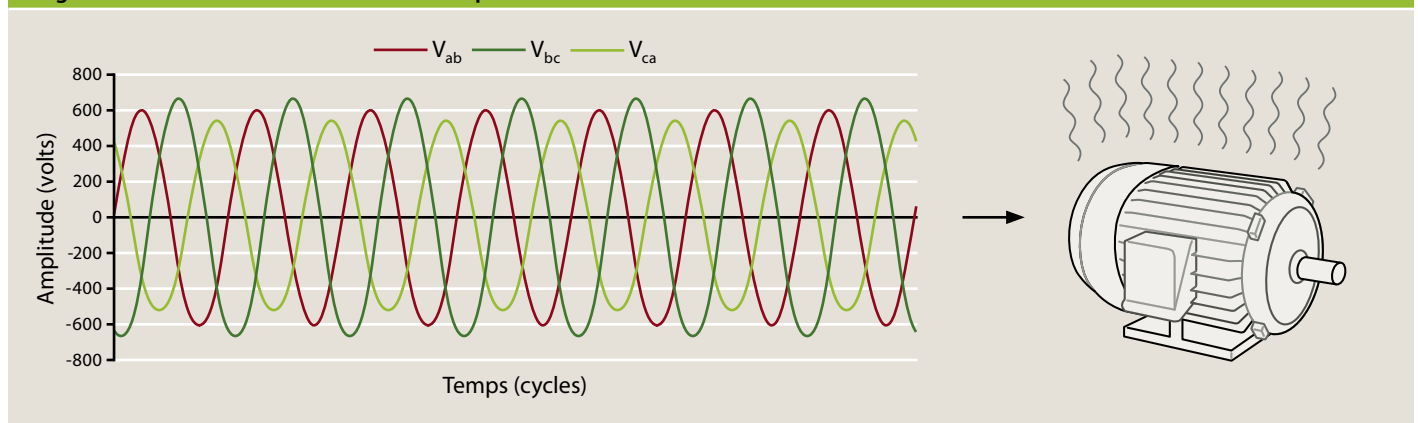
Figure 1 : Forme d'onde illustrant un déséquilibre de tension
