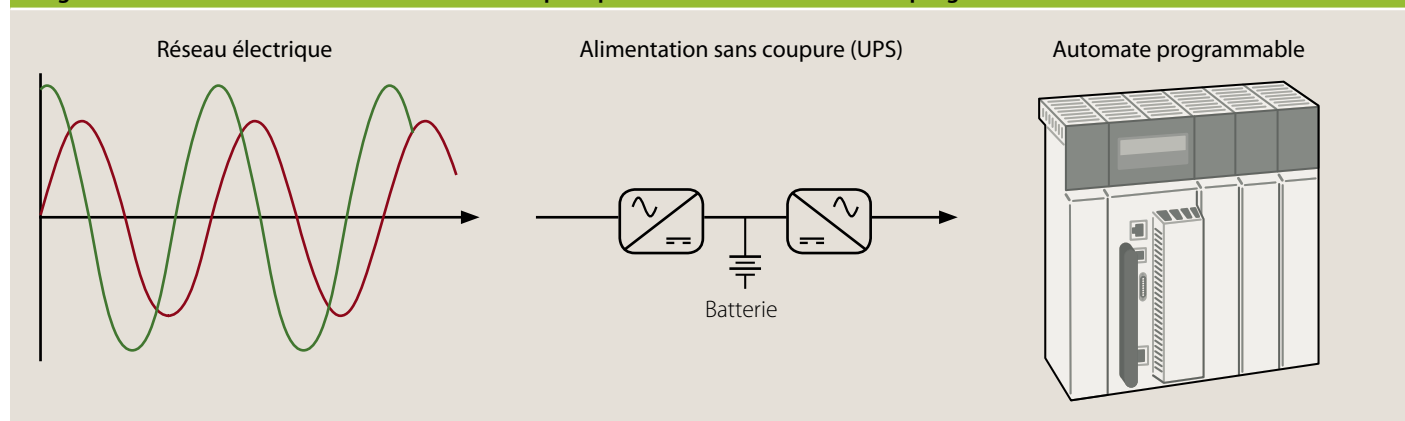
Figure 1 : Utilisation d'une alimentation sans coupure pour immuniser un automate programmable
