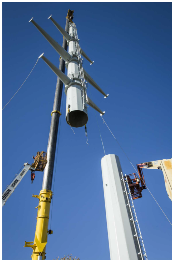
Montage d'un pylône tubulaire
