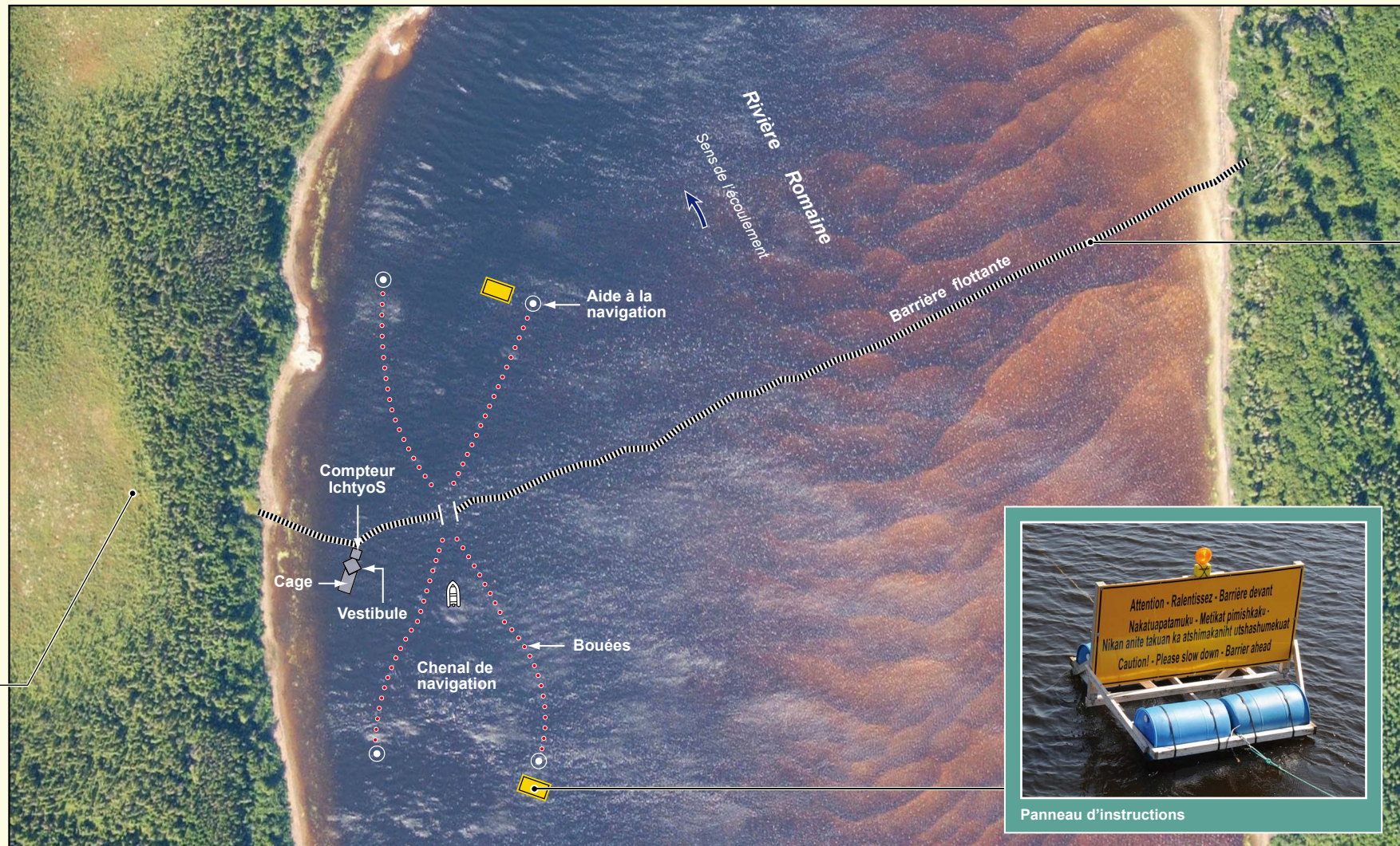
Représentation schématique du système de comptage IchtyoS
