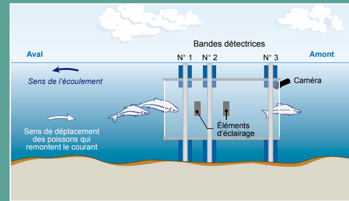
Représentation schématique du système de comptage IchtyoS
