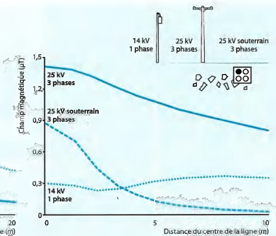
CHAMP MAGNÉTIQUE GÉNÉRÉ PAR LES LIGNES DE DISTRIBUTION (μT)
