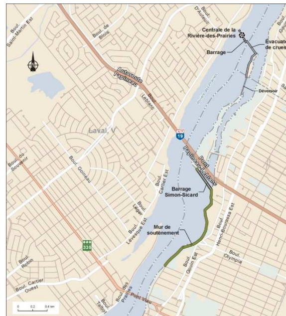
Localisation du mur de soutènement
