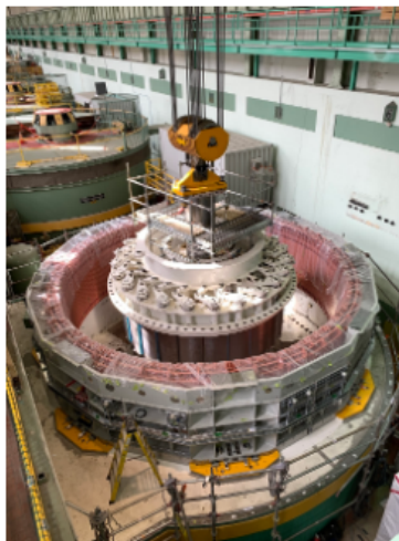
Mars 2022 – Mise en place de l'ensemble arbre, roue et distributeur à l'intérieur du puits turbine
