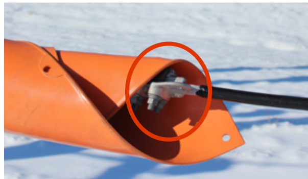
Partie de conducteur laissée à nu par le protecteur
