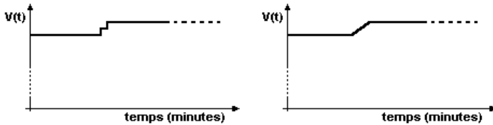
Figure 9 – Variations de tension en doubles échelons et en rampes
