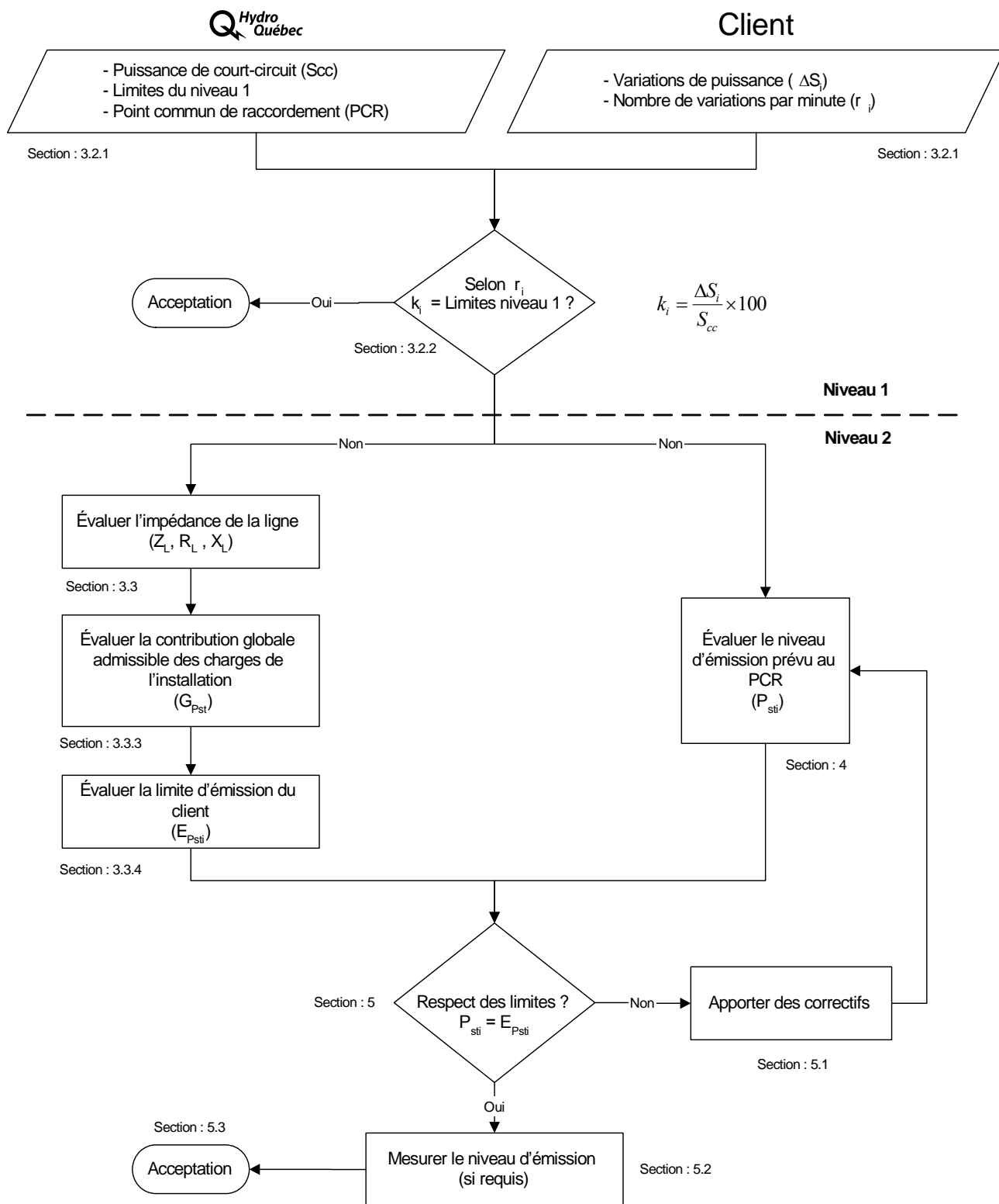
Figure 4 – Processus d'évaluation du papillotement
